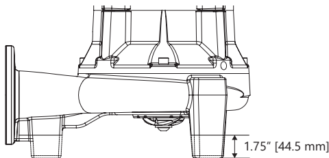
Figura 3. Punto de corte para bombas de 10 a 15 hp
